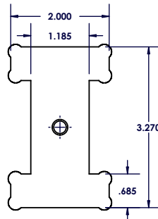
VF2-TP-CP TAPPED
