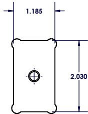
VF2-S-CP SMOOTH
